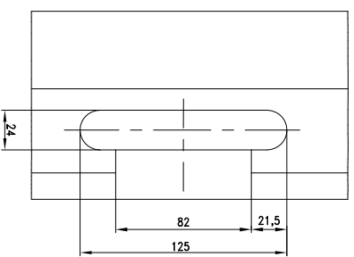
Frezing in het kozijn voor suurtrom automatisch
