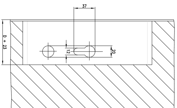
Frezing voor de Hoofdslotkast
