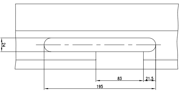
Frezing in kozijn voor sluitkom hoofdslot
