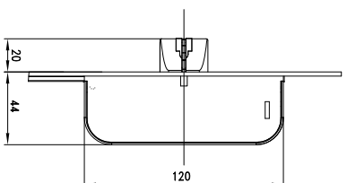
Bijzetslotkast met automatisch schoot
