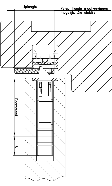
Doorsnede deur en kozijn
