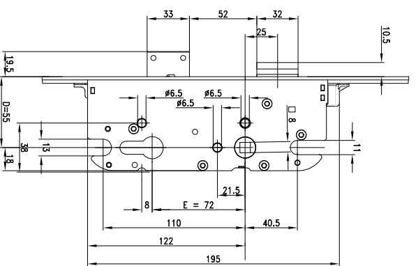
Maatvoering hoofdslotkast
