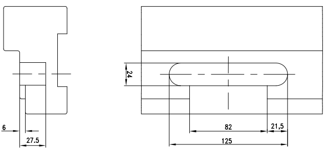
Frezing in het kozijn voor sluitkom automatische schoot
