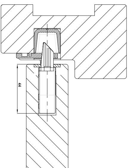
Automatisch schoot
