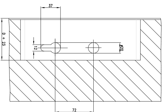
Frezing voor de hoofdslotkast
