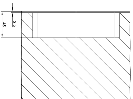
Frezing voor bijzetslotkast voor automatisch schoot
