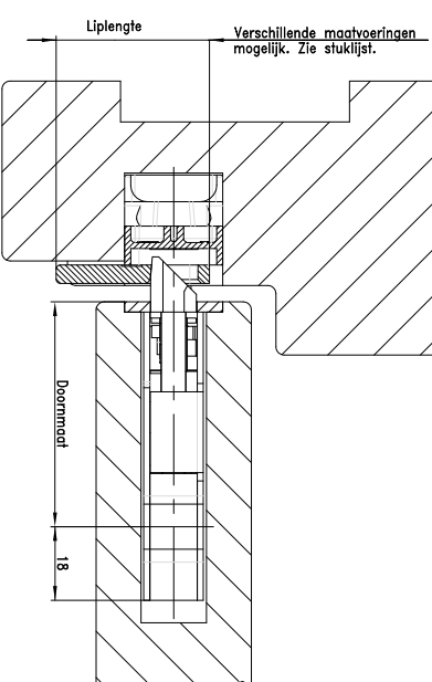
Doorsnede deur en kozijn
