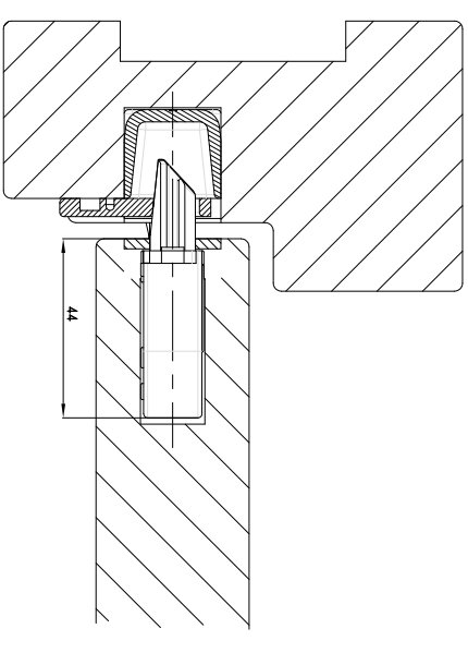
Automatische schoot
