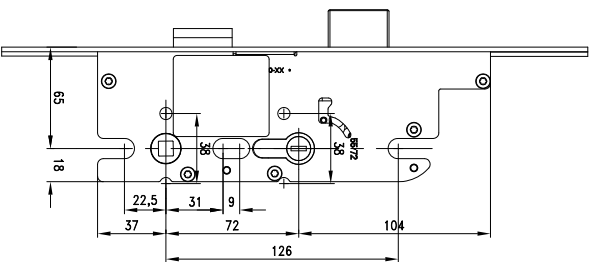
Maatvoering hoofdslotkast
