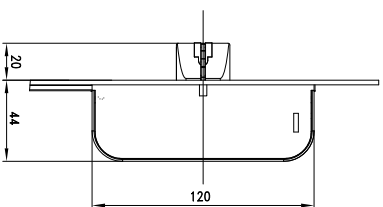
Bijzetslotkast met automatische schoot
