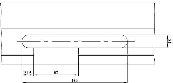
Frezing in kozijn voor suurtrom hoofdslot
