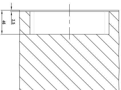
Frezing voor bijzetslotkast voor automatische schoot
