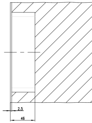
Frezing voor bijzet slotkast voor sluithaak
